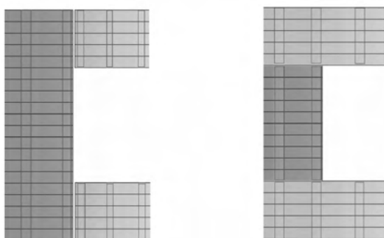
Pavyzdys: Deformacinės siūlės aplink lango angą (plieninis karkasas)
